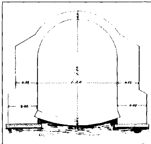
Dwarsdoorsnede van de geplande duiker in de Grote Aa, uit 1857 (coll. GAZ).
