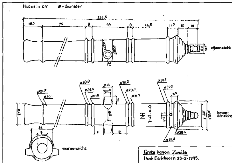
Bouwtekening van het grootste kanon door Henk Eenkhoorn, d.d. 23-2-1995.
