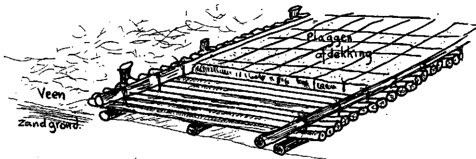
fig.2 Voorstelling van een brugge; tekening van de auteur.
