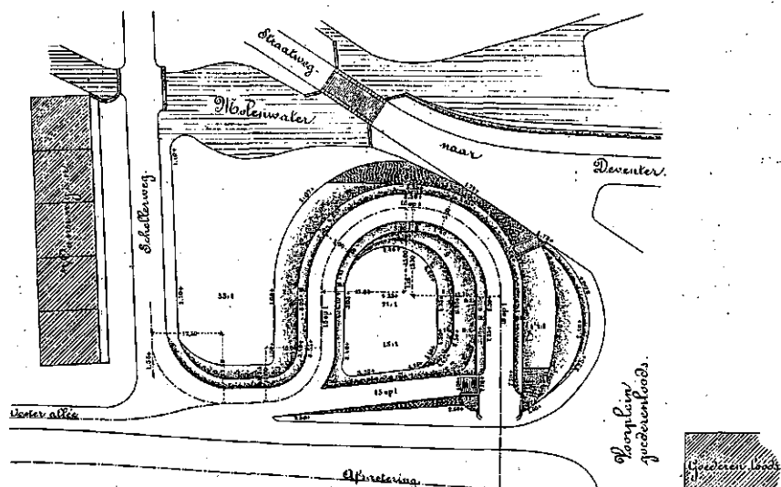
43. Fragment van bestektekening behorende tot Bestek 799, aanbesteed 1 juni 1881, 'wegens het maken van eenige grondwerken, gebouwen, bestratingen, overgangs, afsluitings- en verdere werken (...)'.
