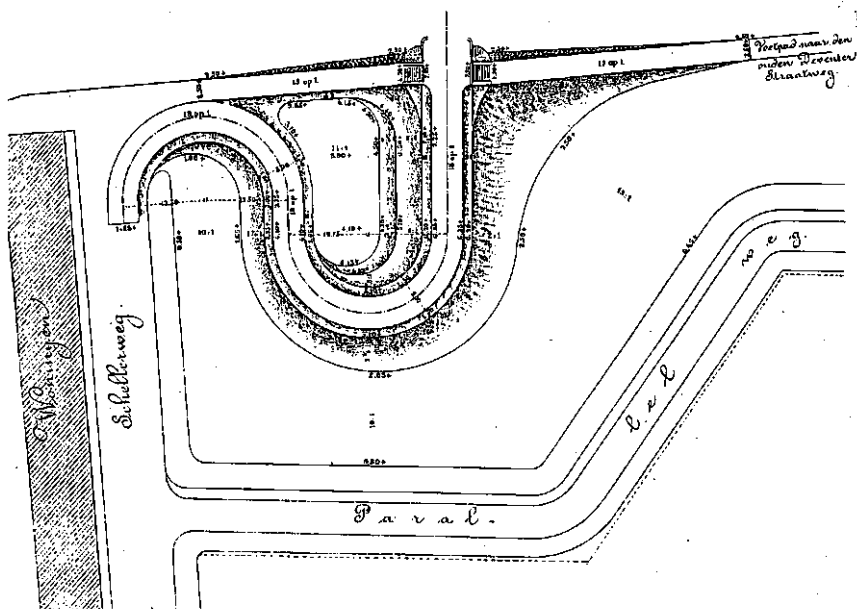
44. De 'aarden toegang' tot de Hoge Brug aan de Schellerzijde. Bestek 799, 1881.
