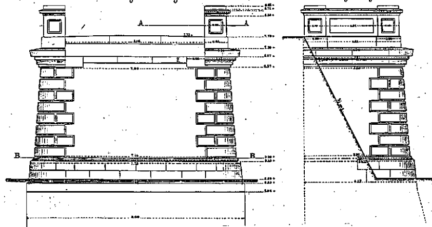
45. Bestek 799 uit 1881. Art. 4: 'De onderbouw voor eene brug over het station bestaat uit twee steenen landhoofden op eene paalfundering en twee steenen voetingen voor tusschensteunpunten, mede op eene paalfundering (...). In de landhoofden is 12\frac{1}{4} m 3 hardsteen en 51 m 3 Noors graniet verwerkt.
