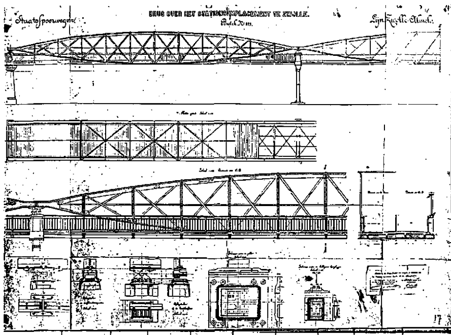
46. Bestektekening van de 'Brug over het stationemplacement te Zwolle'. Staatsspoorwegen, lijn Zwolle Almelo. Bestek 833.
