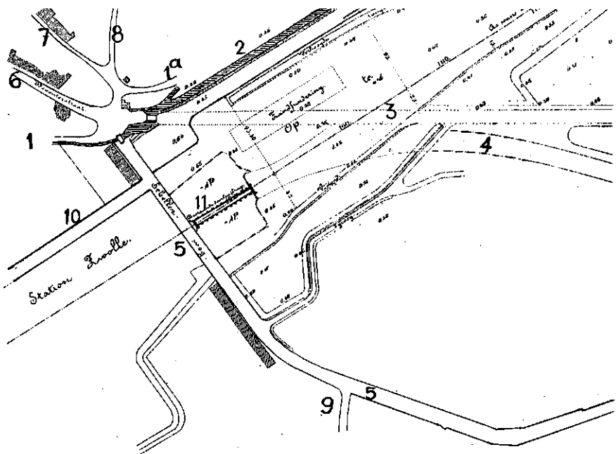
42. Fragment van bestektekening bij Bestek 751 tot uitbreiding van het emplacement (aanbesteed 12 mei 1880).
