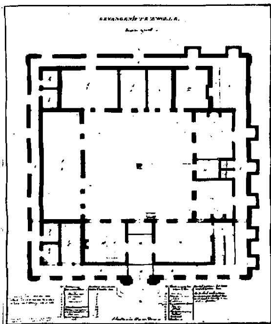
Plattegrond van de parterre van het Huis van Bewaring te Zwolle in 1836 (RAD, kaartencollectie).
